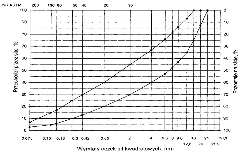
Rys. 2. Krzywe graniczne uziarnienia mieszanek mineralnych BA od 0 do 20 mm do warstwy wiążącej, wyrównawczej i wzmacniającej nawierzchni drogi o obciążeniu ruchem KR1 lub KR2
